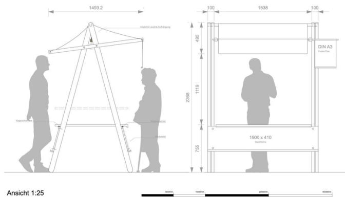
Ansicht 1:25
